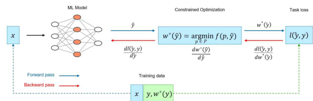
〈그림 2〉 DFL 프레임워크 [2]
